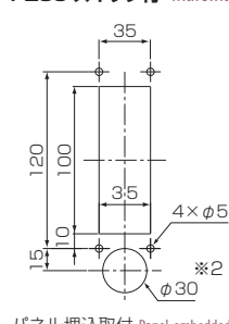
パネル埋込取付 Panel-embedded
