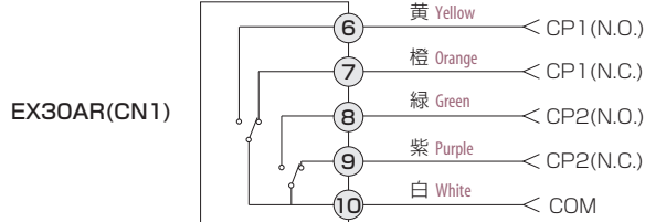
比較出力の接続 Connecting comparative output
