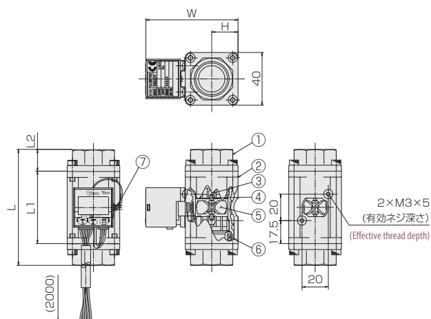
TP-HP バルブ無し With no valve
