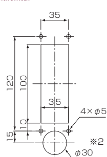
パネル埋込取付 Panel-embedded
