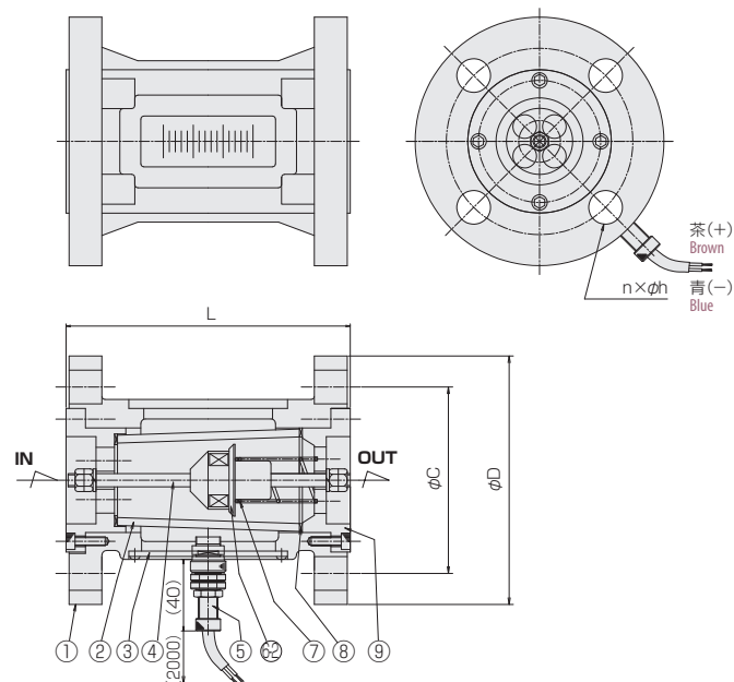
リードスイッチ付 with reed switch
