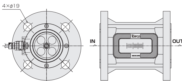
リードスイッチ付 With reed switch
