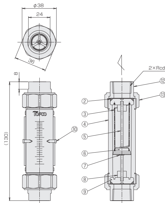
ユニオンフィッティングタイプ Union fitting type
