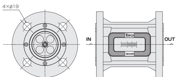
スイッチなし With no switch
