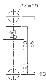
パネル前面取付 Panel-mounted
