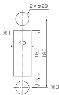
パネル前面取付 Panel-mounted
