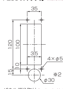
パネル埋込取付 Panel-embedded
